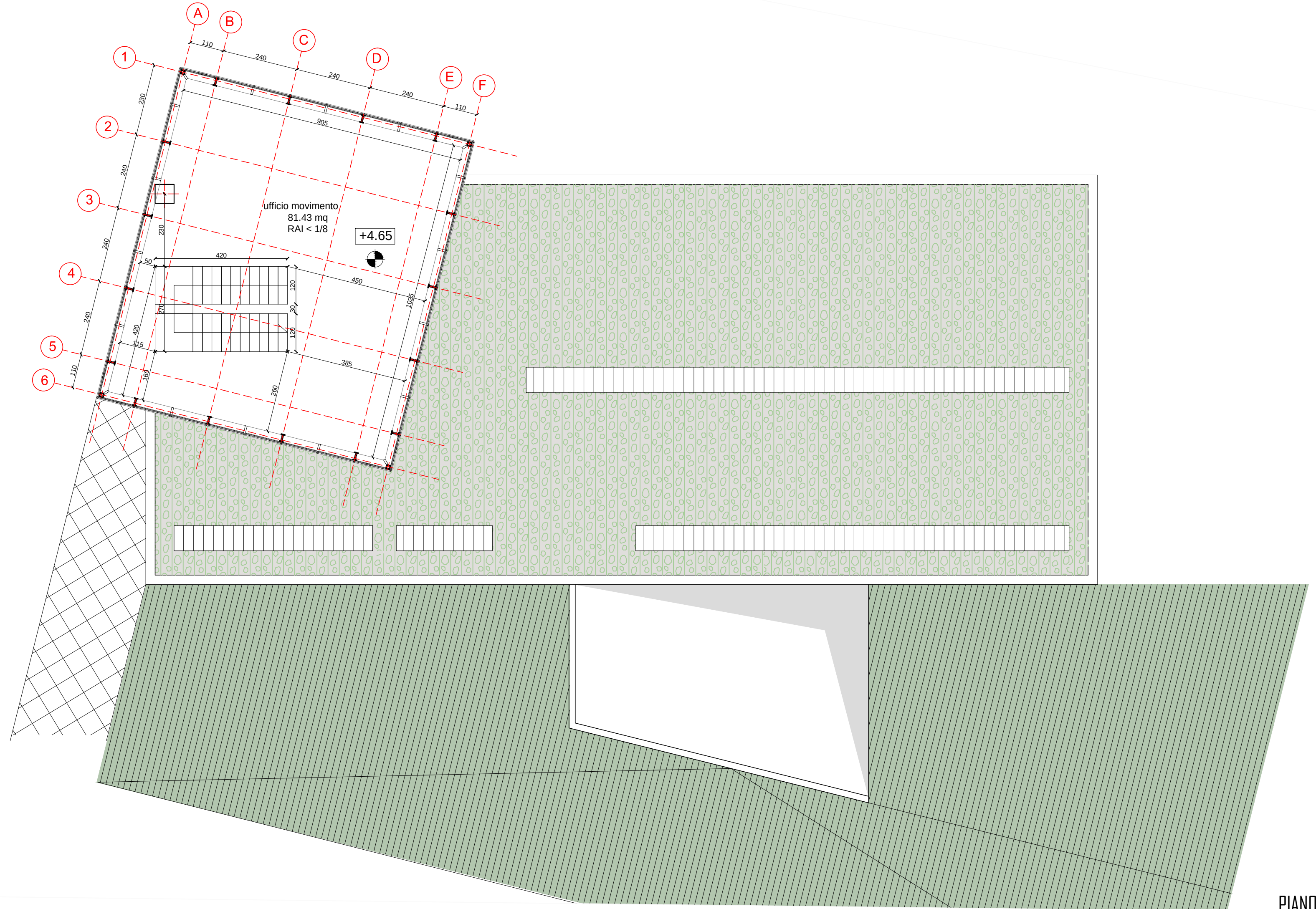
PIANO PRIMO
